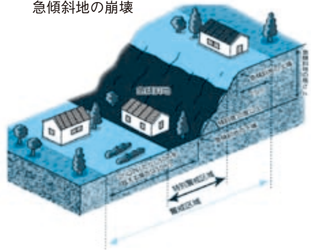
急傾斜地の崩壊
